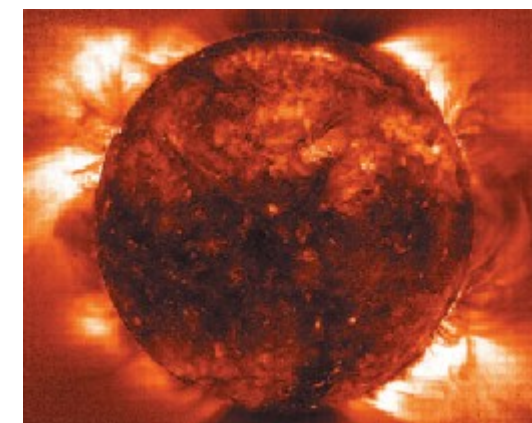
Le Soleil vu en rayons X ; ici seules les régions extrêmement chaudes de la couronne (million de degrés) émettent de la lumière. Satellite SOHO © J. P. Delaboudinière et Consortium EIT
