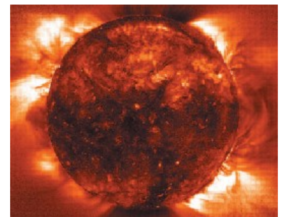
Le Soleil vu en rayons X ; ici seules les régions extrêmement chaudes de la couronne (million de degrés) émettent de la lumière. Satellite SOHO © J. P. Delaboudinière et Consortium EIT
