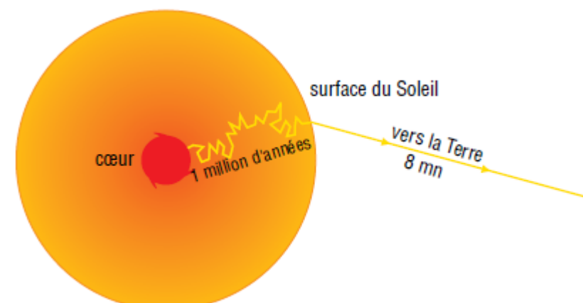
Le chemin de la lumière solaire.
