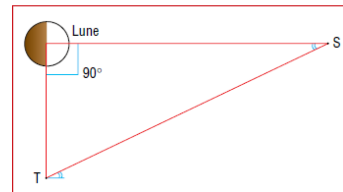
Géométrie du système Soleil – Terre – Lune précisément au premier quartier.
