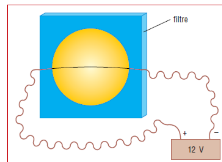
La surface du Soleil a une température plus élevée que celle d'un fil porté au blanc.
